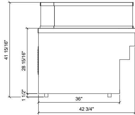
2 VUE DE CÔTÉ 1 1/2" = 1'-0"
