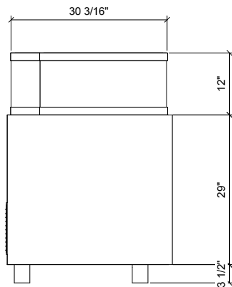
② VUE DE CÔTÉ 1 1/2" = 1'-0"
