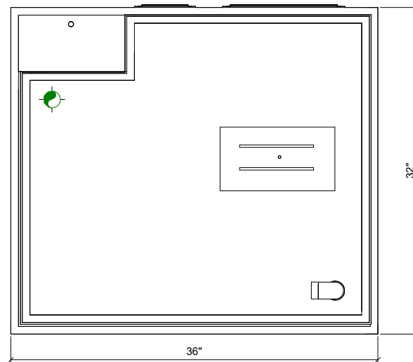
④ VUE DE HAUT 3" = 1'-0"
