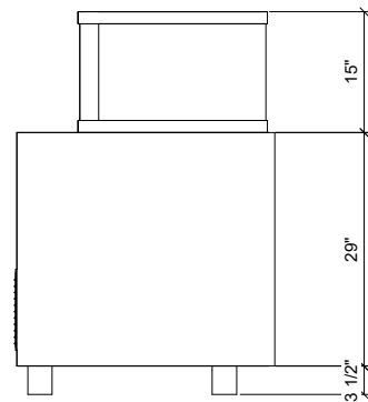
② VUE DE CÔTÉ 1 1/2" = 1'-0"
